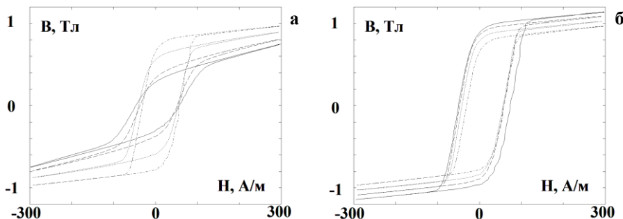
Рис. 7. Петли гистерезиса аморфных лент состава \text{Fe}_{64}\text{Co}_{21}\text{B}_{15} , прошедших термомагнитную обработку при T_{pre}=250^\circ\text{C} в процессе цикла «нагрев-охлаждение». а – нагрев, б – охлаждение. Температура нагрева T : — 20^\circ\text{C} — 200^\circ\text{C} ..... 260^\circ\text{C} — · — 290^\circ\text{C} .
