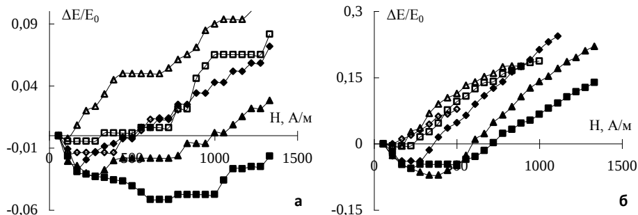
Рис. 10. Полевые зависимости \Delta E -эффекта аморфных проволок состава \text{Fe}_{75}\text{Si}_{10}\text{B}_{15} , прошедших термомагнитную обработку при температурах T_{pre} : а - T_{pre}=370^\circ\text{C} , б - T_{pre}=420^\circ\text{C} . Нагрев образца. Температура T : ■ - T=30^\circ\text{C} , ▲ - T=90^\circ\text{C} , ◆ - T=150^\circ\text{C} , □ - T=210^\circ\text{C} , △ - T=240^\circ\text{C} .
