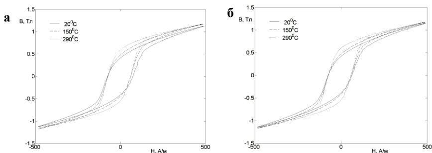
Рис. 12. Петли гистерезиса аморфных проволок состава \text{Fe}_{75}\text{Si}_{10}\text{B}_{15} , прошедших термомагнитную обработку при T_{pre}=420^\circ\text{C} . (а) - нагрев, (б) - охлаждение.
