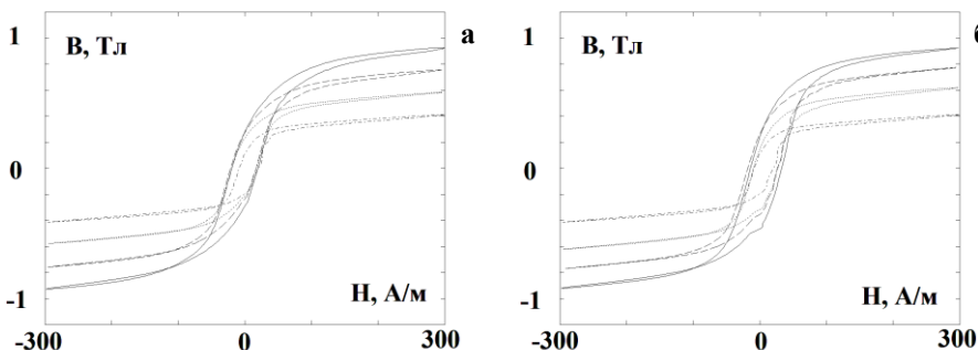
Рис. 3. Петли гистерезиса аморфных лент состава \text{Fe}_{67}\text{Co}_{10}\text{Cr}_3\text{Si}_{15}\text{B}_5 , прошедших термомагнитную обработку при T_{\text{pre}}=370^\circ\text{C} в процессе цикла «нагрев-охлаждение». а - нагрев; б - охлаждение. Температура нагрева T : — 20^\circ\text{C} - - 200^\circ\text{C} ..... 260^\circ\text{C} - · - 290^\circ\text{C} .
