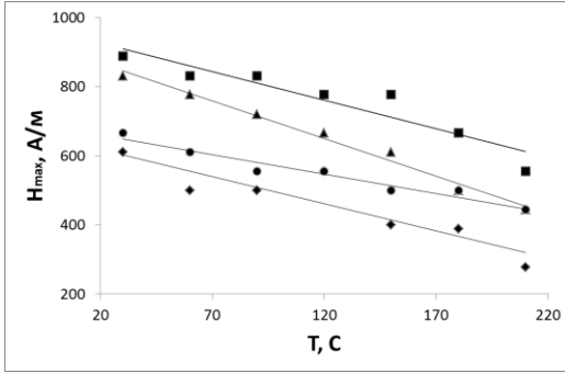
Рис. 6. Зависимости H_{max}(T) , полученные при нагреве аморфных металлических лент состава \text{Fe}_{64}\text{Co}_{21}\text{B}_{15} , прошедших термомагнитную обработку при температурах T_{pre} :
